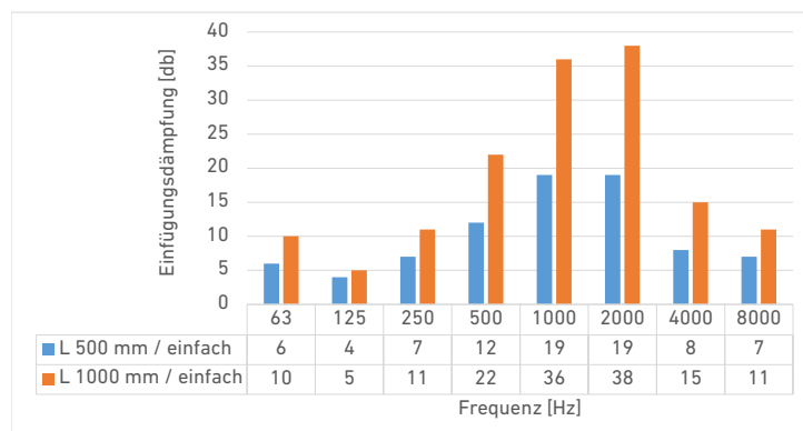
Einfügungsdämpfung
